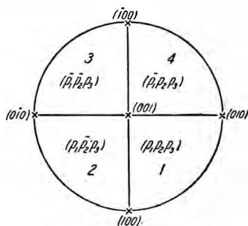
Ромбическая симметрия
