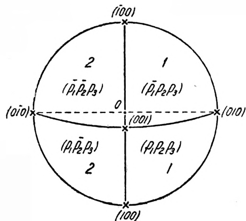
Моноклинные симметрия
