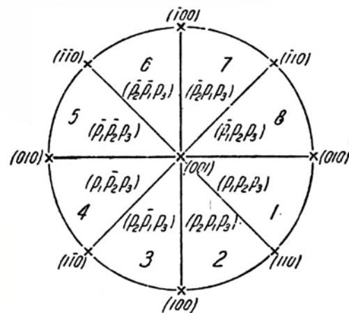
Тетрагональная симметрия
