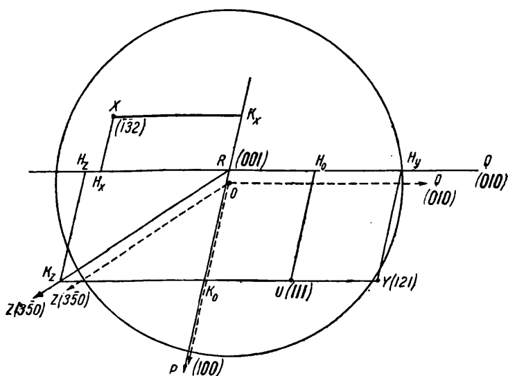
З. Через точку R проводим прямую RZ , параллельную радиусу OZ , на котором в бесконечности лежит проекция грани Z . На прямой RZ берем любую точку K . По формуле (16) имеем:
