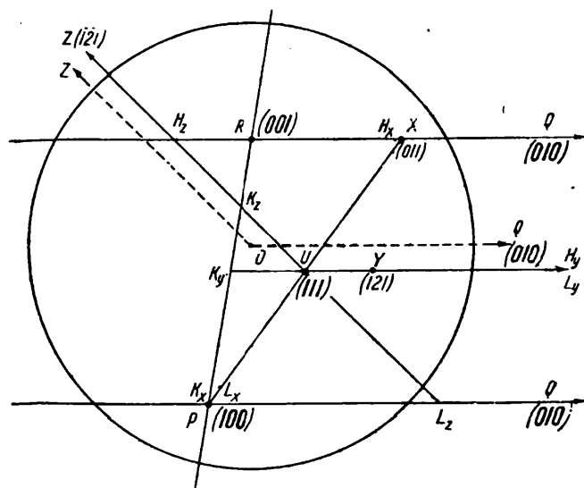
§ 5. Две из основных граней параллельны оси проекций
