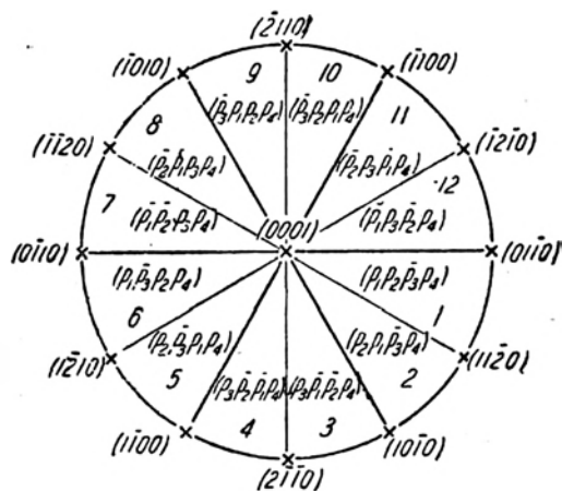
Гексагональная симметрия
