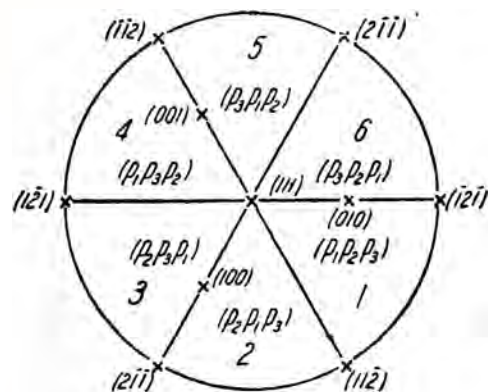
Тригональная (ромбоэдрическая) симметрия
